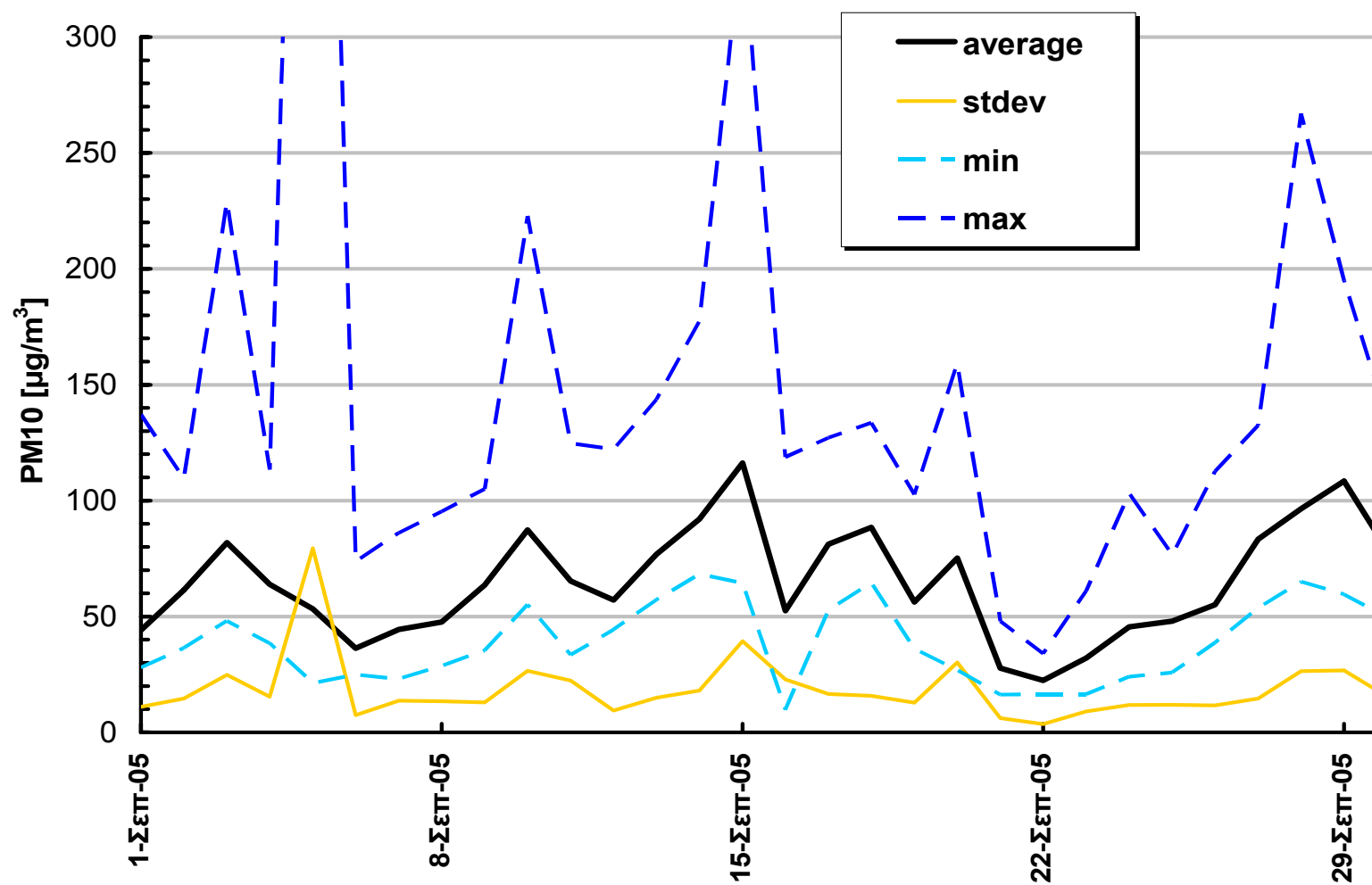
Εικόνα 1 Μηνιαία διακύμανση ημερησίων τιμών (Σεπτέμβριος 2005)
