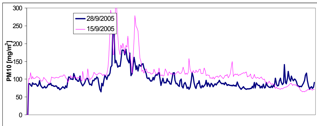
Εικόνα 2 Σύγκριση ημερήσιας διακύμανσης συγκεντρώσεων PM10 (δύο καθαρές με δύο βεβαρημένες μέρες) .
